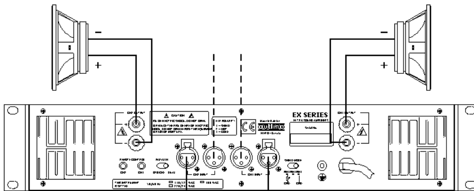
COLLEGAMENTO PARALLELO PARALLEL CONNECTION ПАРАЛЛЕЛЬНОЕ ПОДКЛЮЧЕНИЕ
